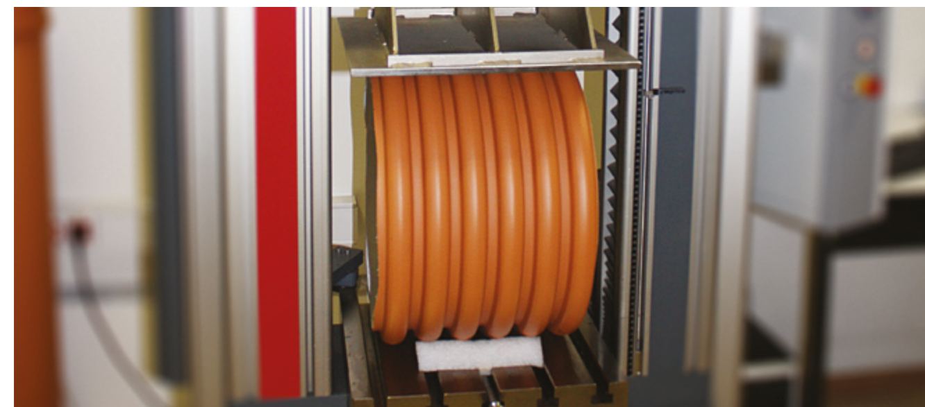
лабораторные испытания трубы Polytron ProKan
